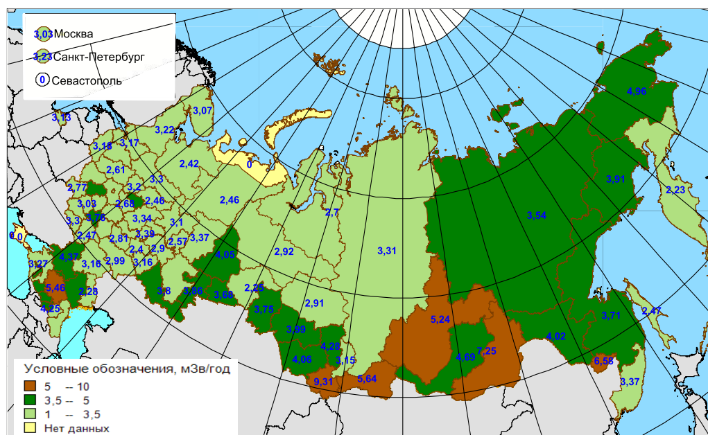
Рис. 41. Средние годовые эффективные дозы облучения населения за счет природных источников, по данным за период 2001–2016 гг.
